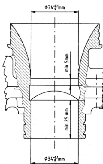
PLAN CARBURATEUR
